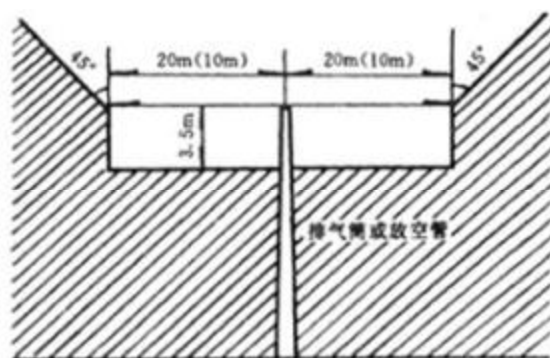
图 5.5.11 可燃气体排气筒、放空管高度示意图
