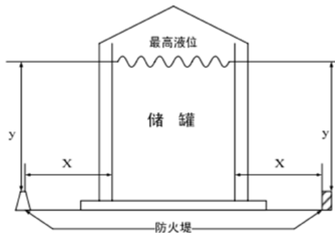
图 6.3.6 单防罐至防火堤内顶角线的距离
